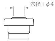
15-415用4φ穴明中栓(被せ)
