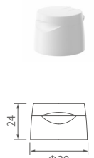
T-40Φ Flip-Top CAP (O/D: Φ6)
