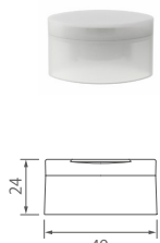
T-40Φ Oval Flip-Top CAP (O/D: Φ1.5 / Φ3)
