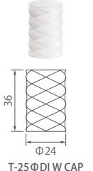
T-25Φ DI W CAP
